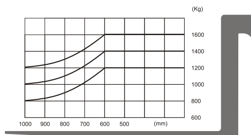
Traglastdiagramm
